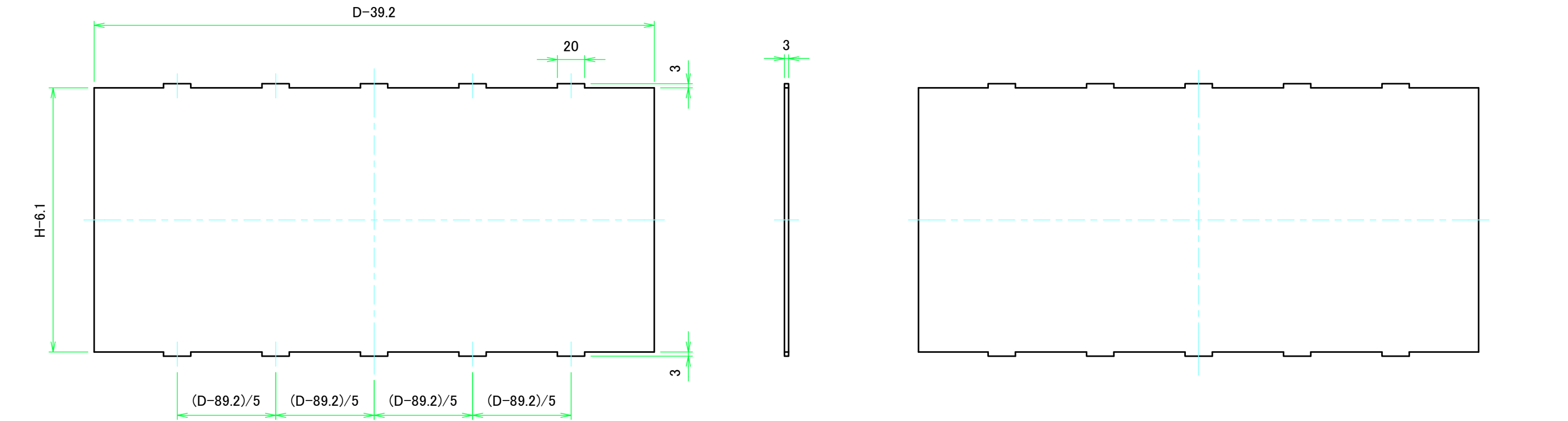
Dパネル1表面 / D Panel 1 Frontside
