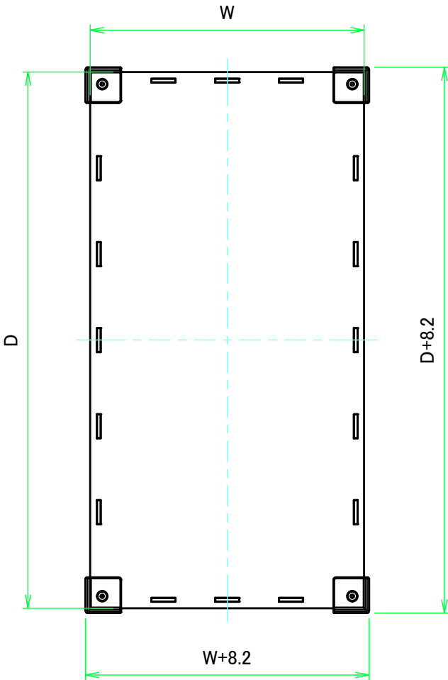
Wパネル1 / W Panel 1
