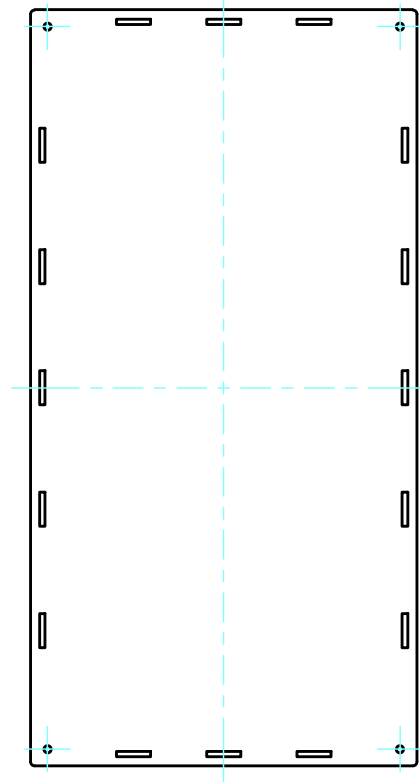
下カバー表面 / Bottom cover Frontside
