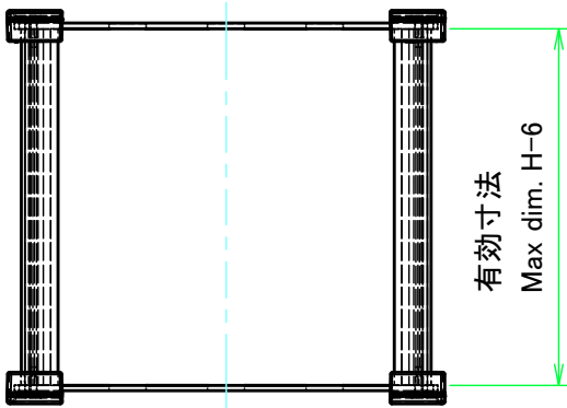
Wパネル1 / W Panel 1
